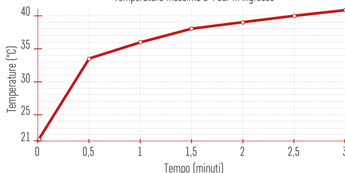
TEMPERATURE Temperatura massima a 4 bar in ingresso
